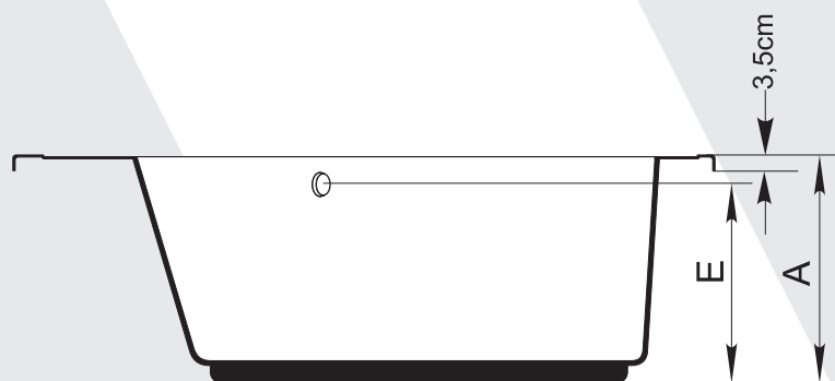
SEÇÃO A - A'
