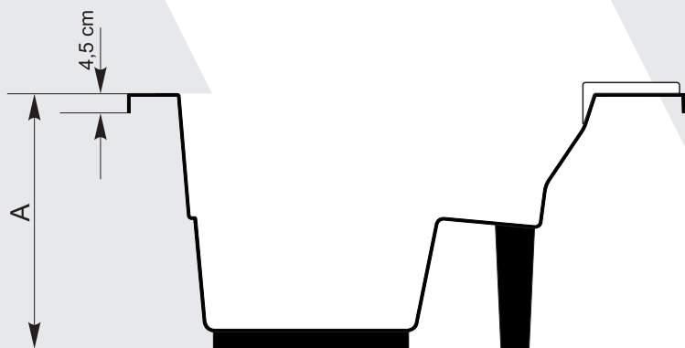
SEÇÃO A - A'
